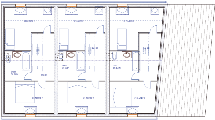
PLAN ETAGE
