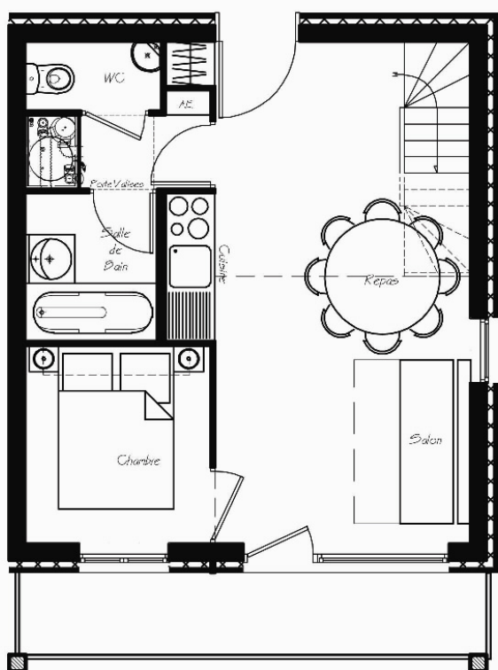
Niveau Entrée
