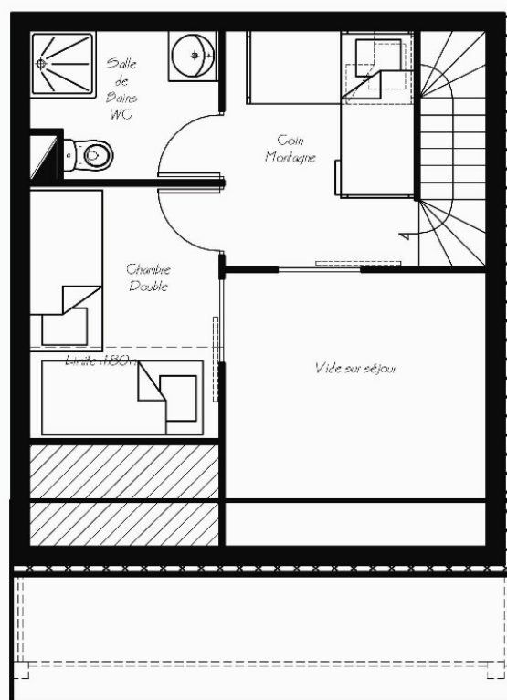
Niveau Mezzanine
