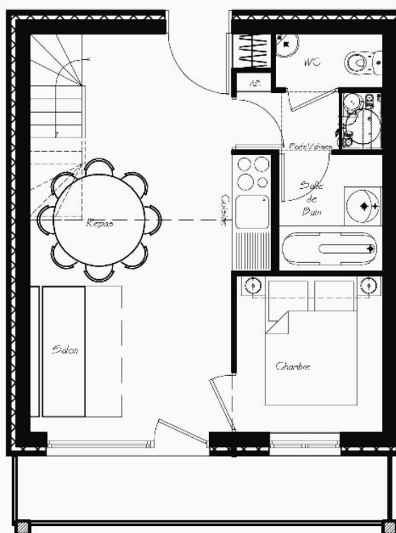
Niveau Entrée
