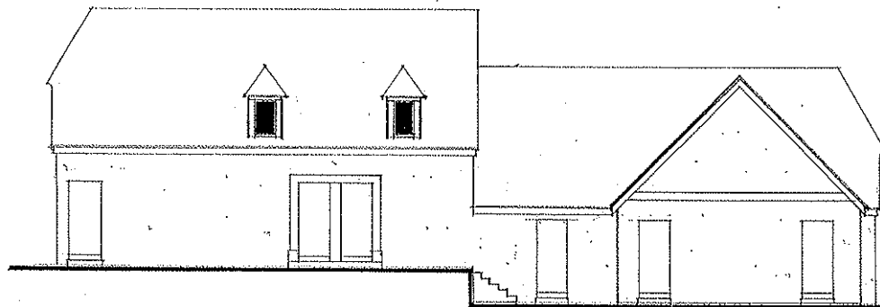
BAT. H NORD EST
