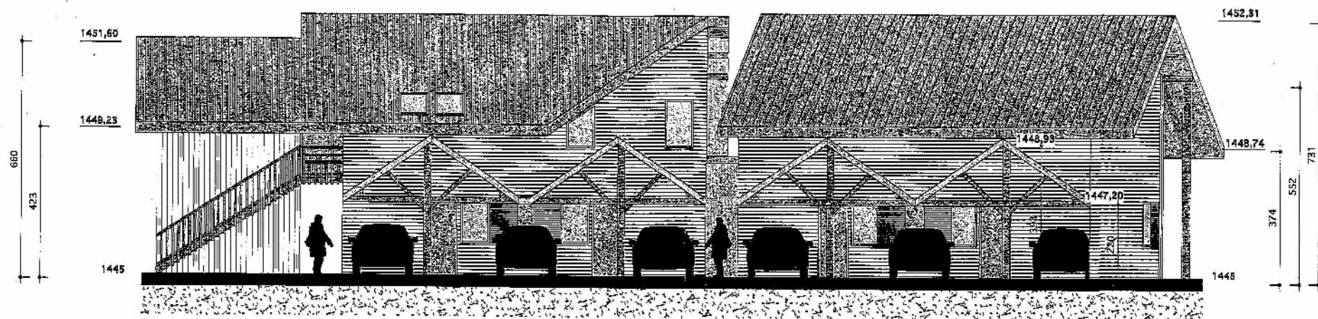
Façade Nord
