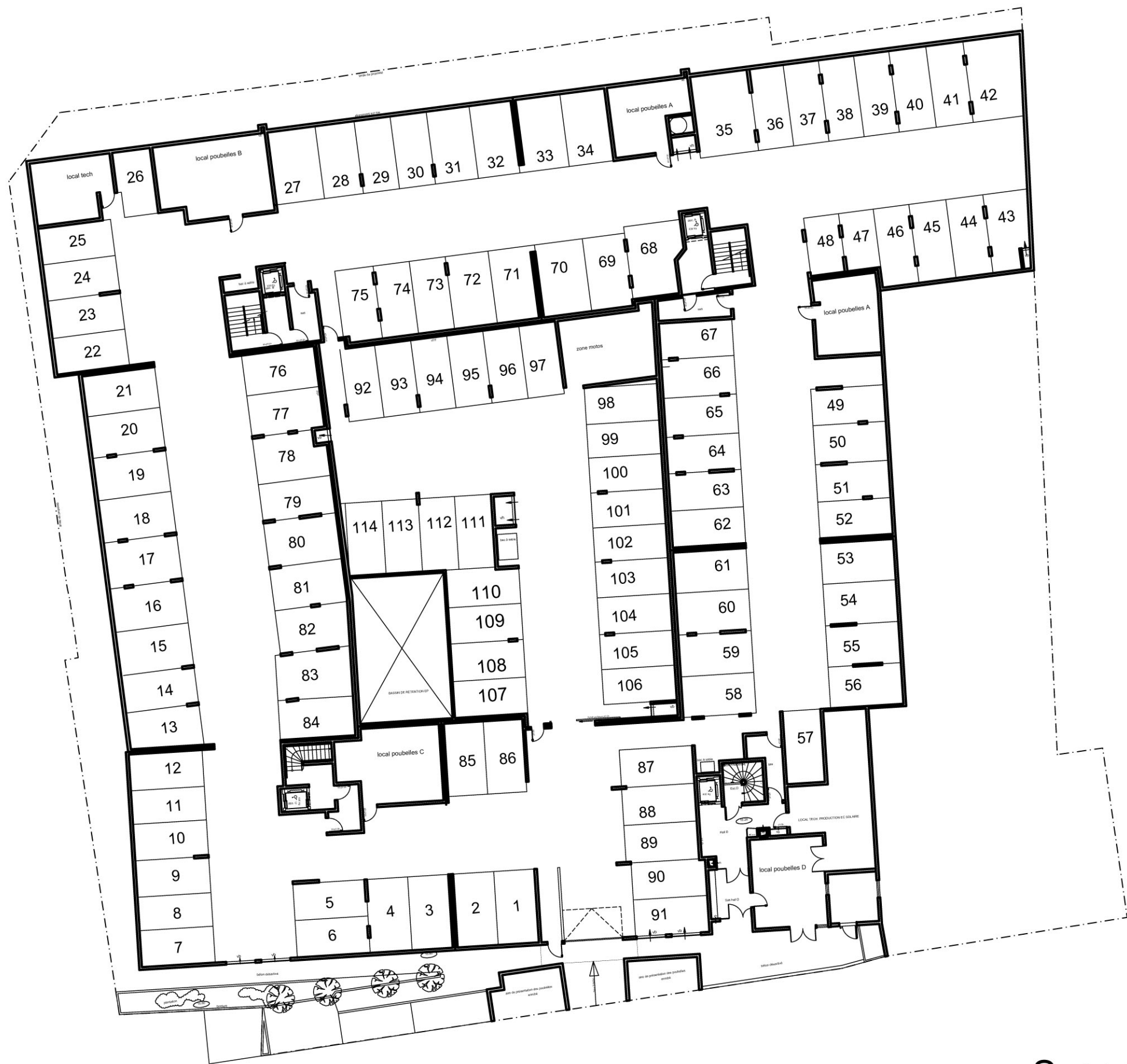
Synoptique du R-1
