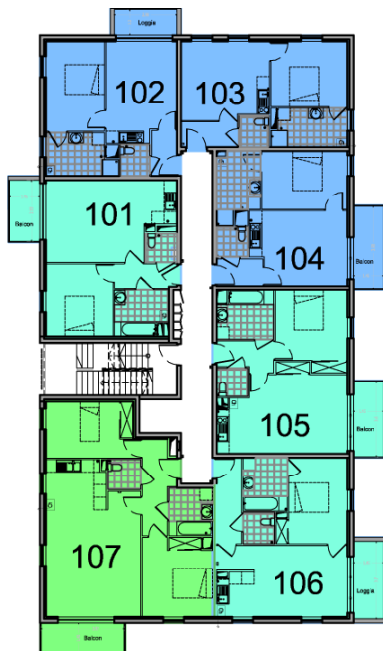
PLAN DU R+1
