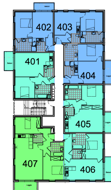
PLAN DU R+4
