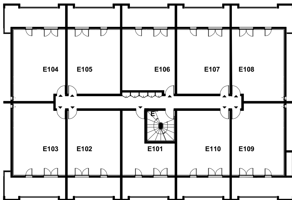
1er ETAGE
