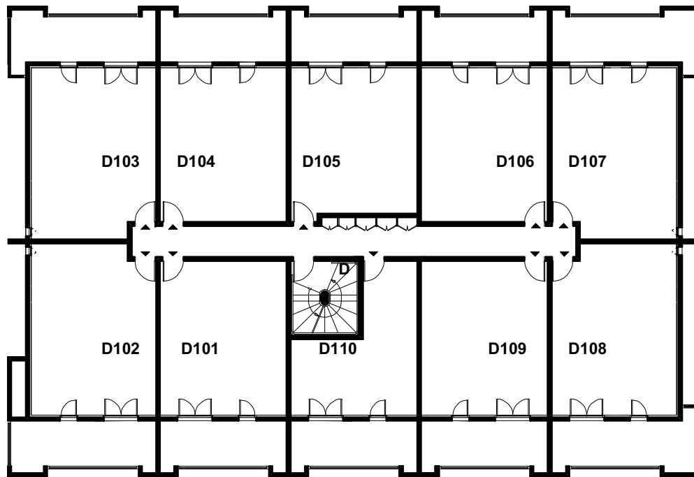
1er ETAGE
