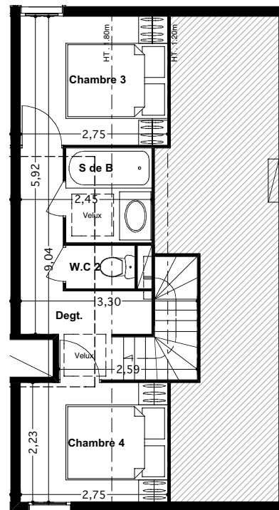
étage
