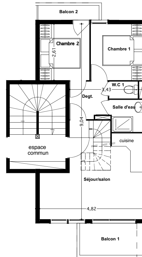
niveau principal
