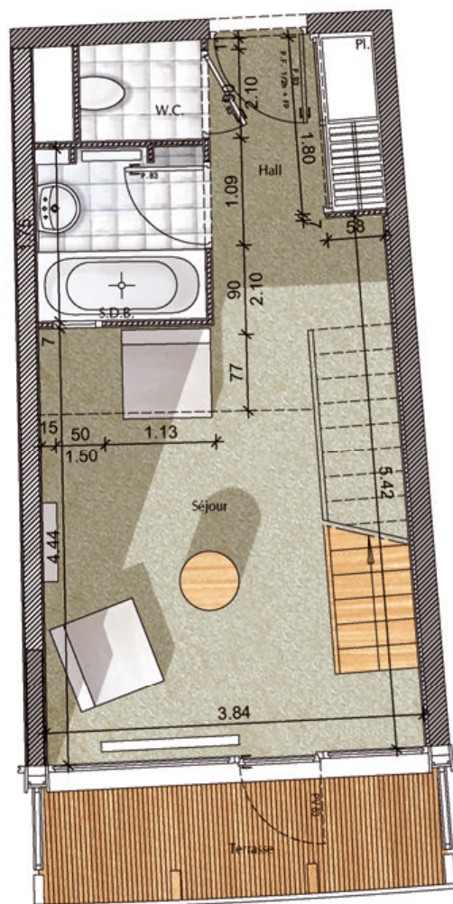
NIVEAU 3
