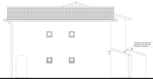
Façade ouest
