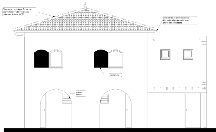
Façade nord
