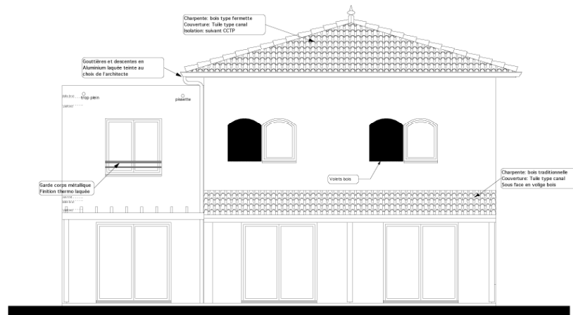
Façade sud
