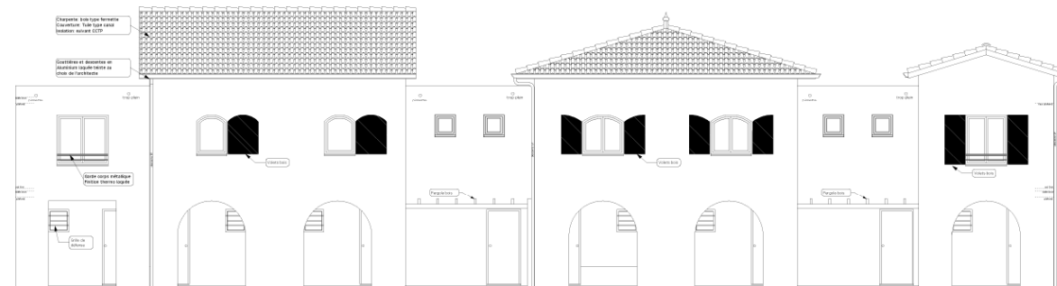
Façade nord
