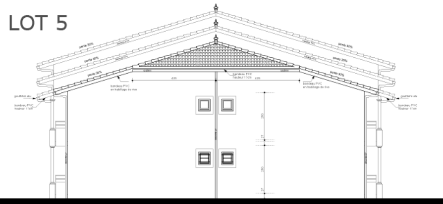
FACADE NORD
