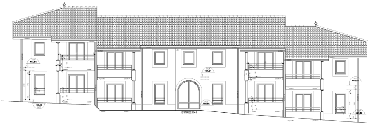
FACADE EST
