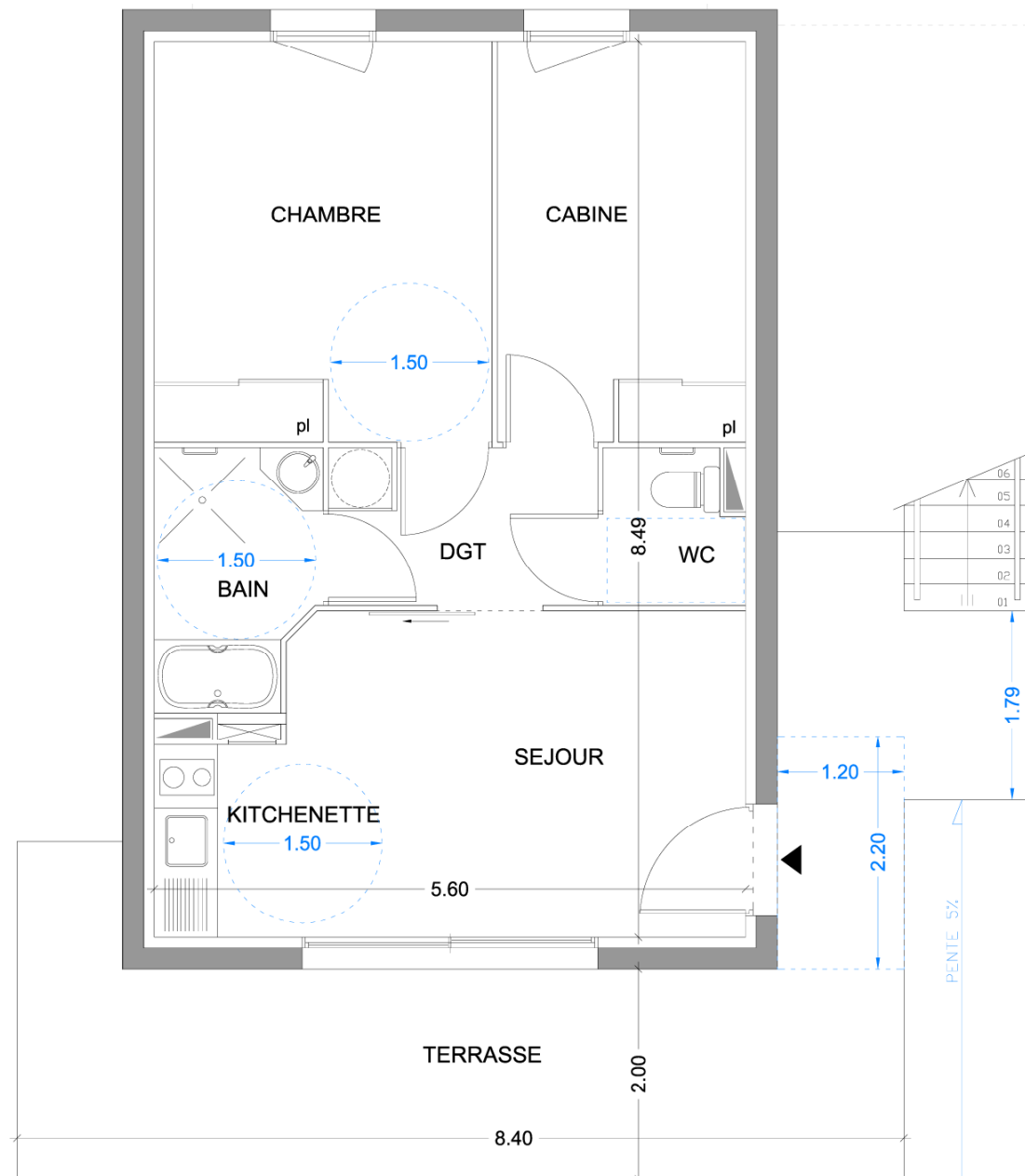
PLAN DU REZ DE CHAUSSEE
