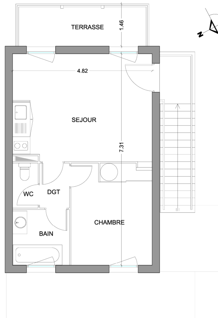
PLAN DU R+1
