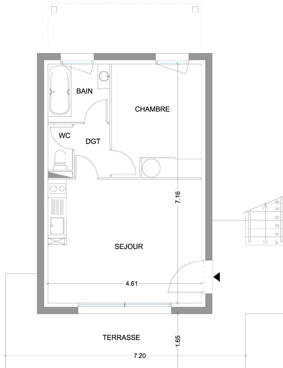
PLAN DU REZ DE CHAUSSEE
