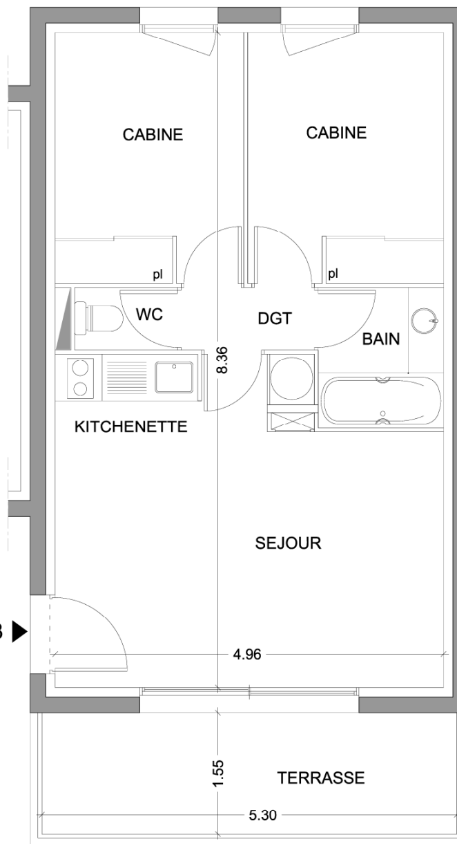
PLAN DU R+1
