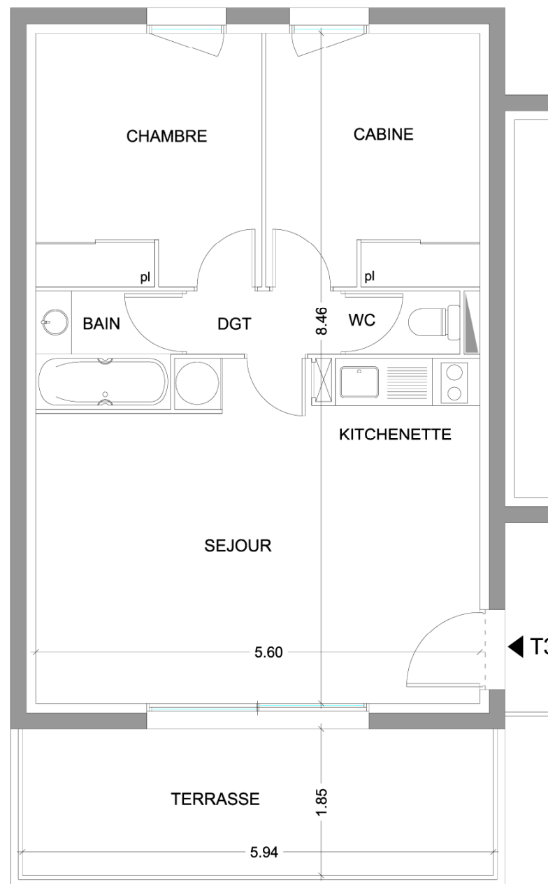
PLAN DU R+1
