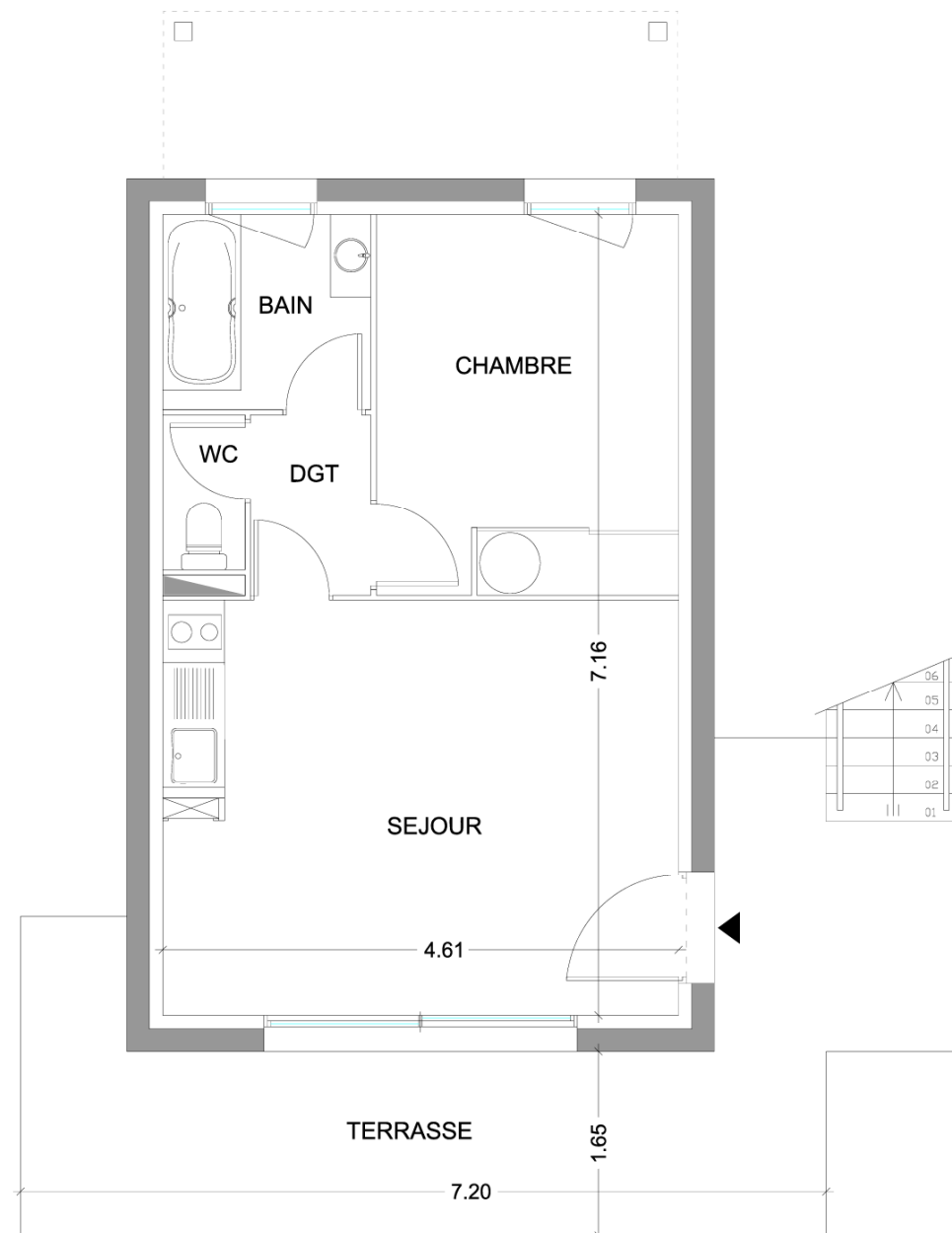
PLAN DU REZ DE CHAUSSEE
