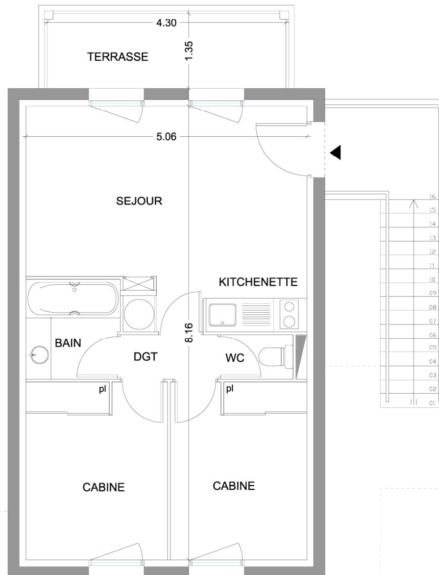
PLAN DU R+1
