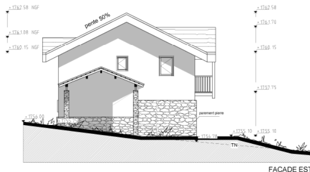
FACADE EST
