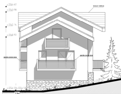
FACADE SUD-OUEST
