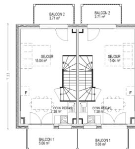
NIVEAU 1
