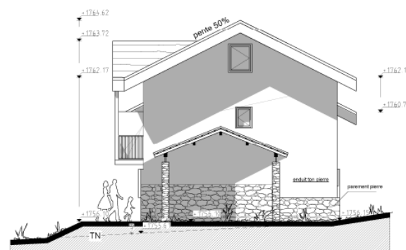
FACADE OUEST
