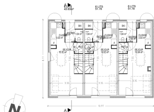
REZ-DE-CHAUSSEE
