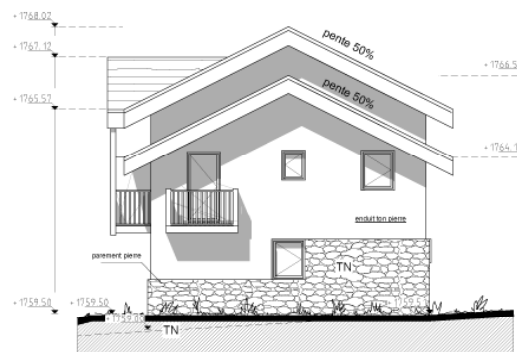
FACADE OUEST
