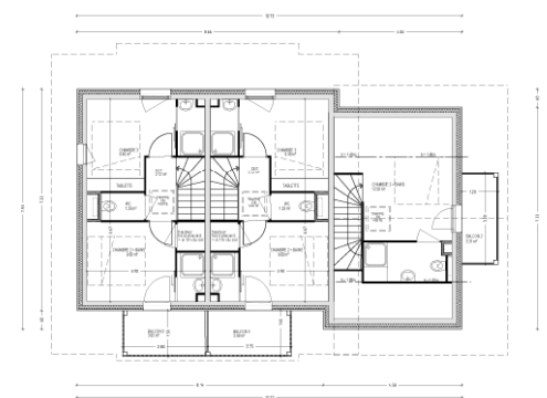
NIVEAU 2
