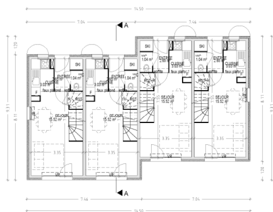
RDC
