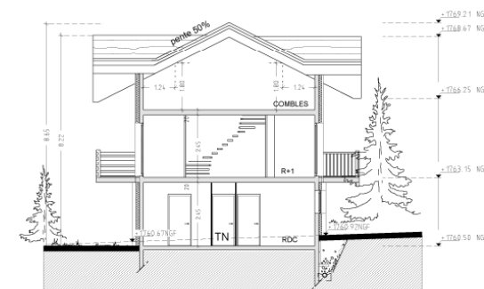
COUPE
