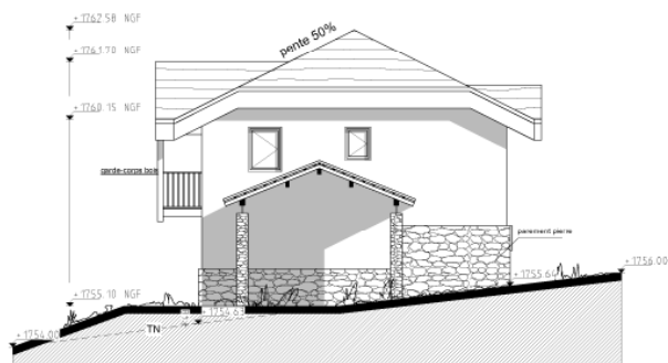
FACADE OUEST
