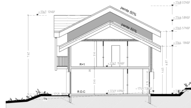
COUPE
