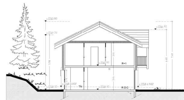
COUPE
