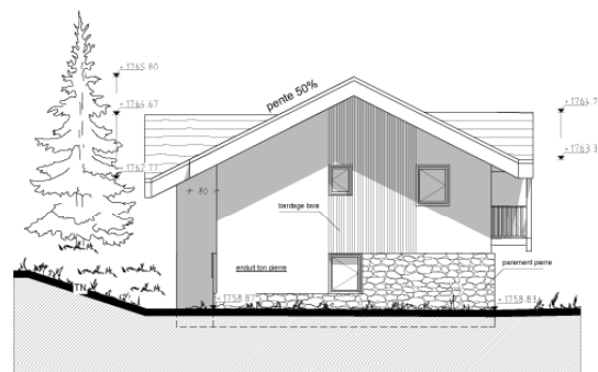
FACADE SUD-EST
