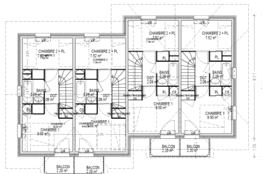
NIVEAU 1
