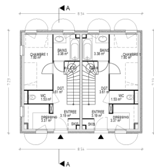
REZ-DE-CHAUSSEE
