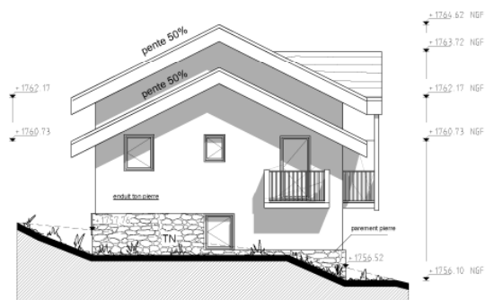
FACADE EST
