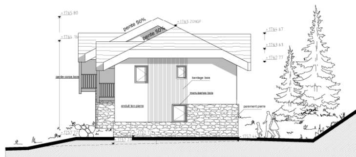
FACADE NORD-OUEST
