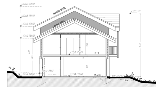
COUPE
