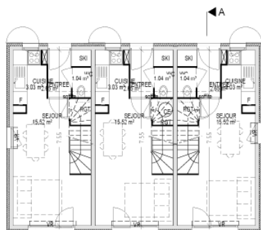
REZ-DE-CHAUSSEE
