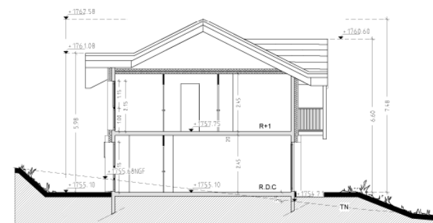
COUPE
