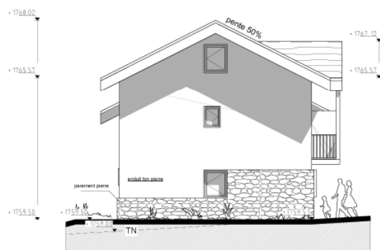
FACADE EST
