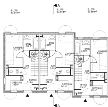
REZ-DE-CHAUSSEE
