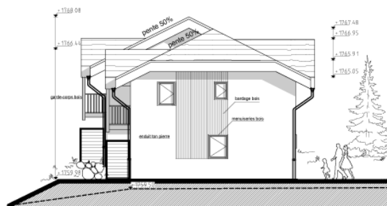
FACADE SUD-OUEST
