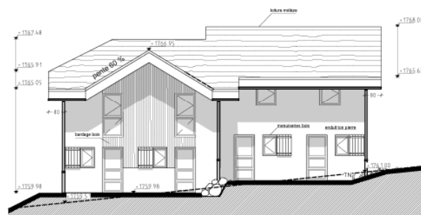
FACADE SUD-EST
