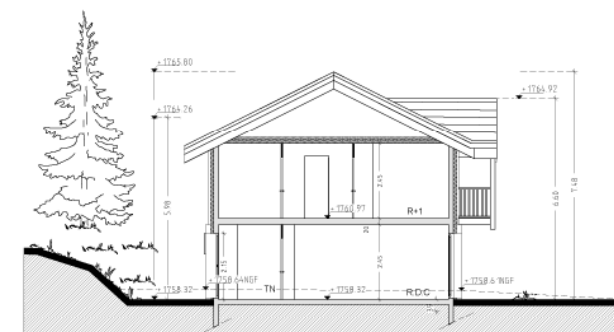
COUPE
