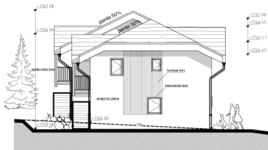
FACADE NORD-EST
