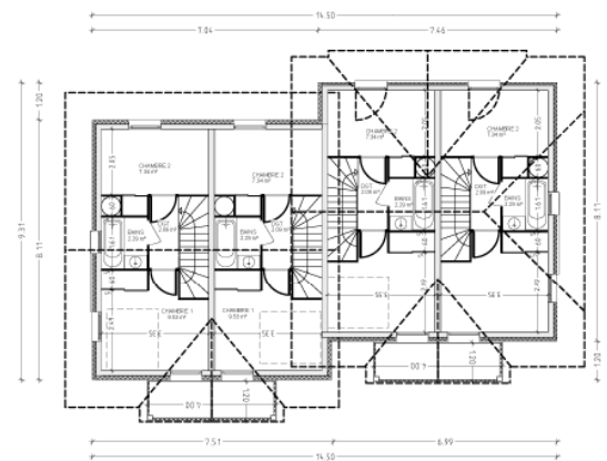
NIVEAU 1
