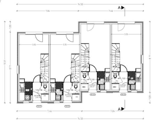
REZ-DE-CHAUSSEE
