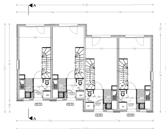
REZ-DE-CHAUSSEE
