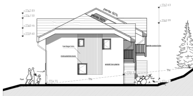
FACADE SUD-OUEST
