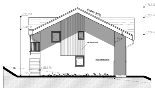
FACADE NORD-EST
