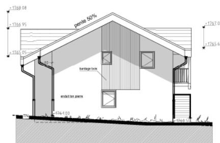
FACADE NORD-EST
