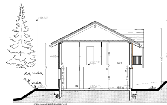
COUPE
