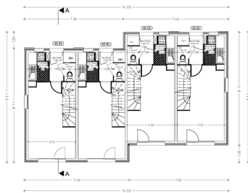
REZ-DE-CHAUSSEE
