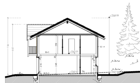
COUPE
