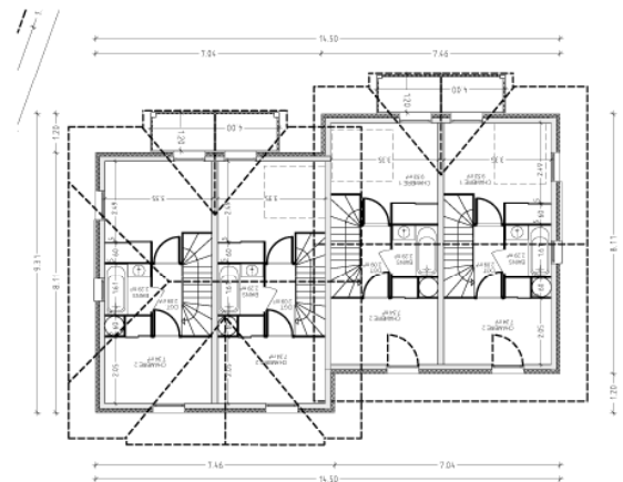
NIVEAU 1
