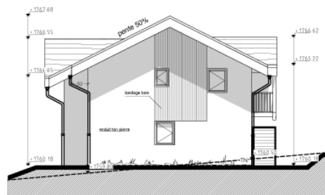
FACADE SUD-OUEST
