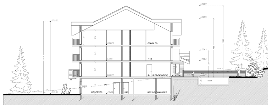
COUPE BB SUR R+3
