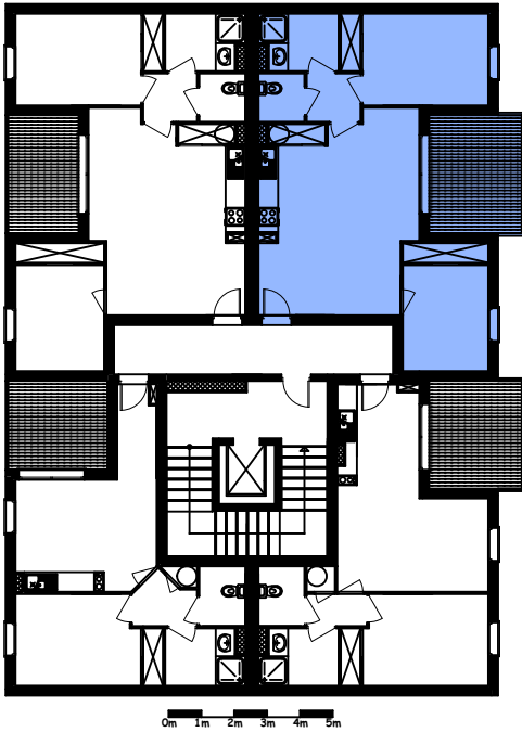
ETAGE 2
