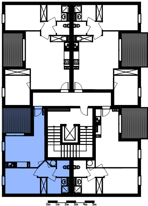
ETAGE 1
