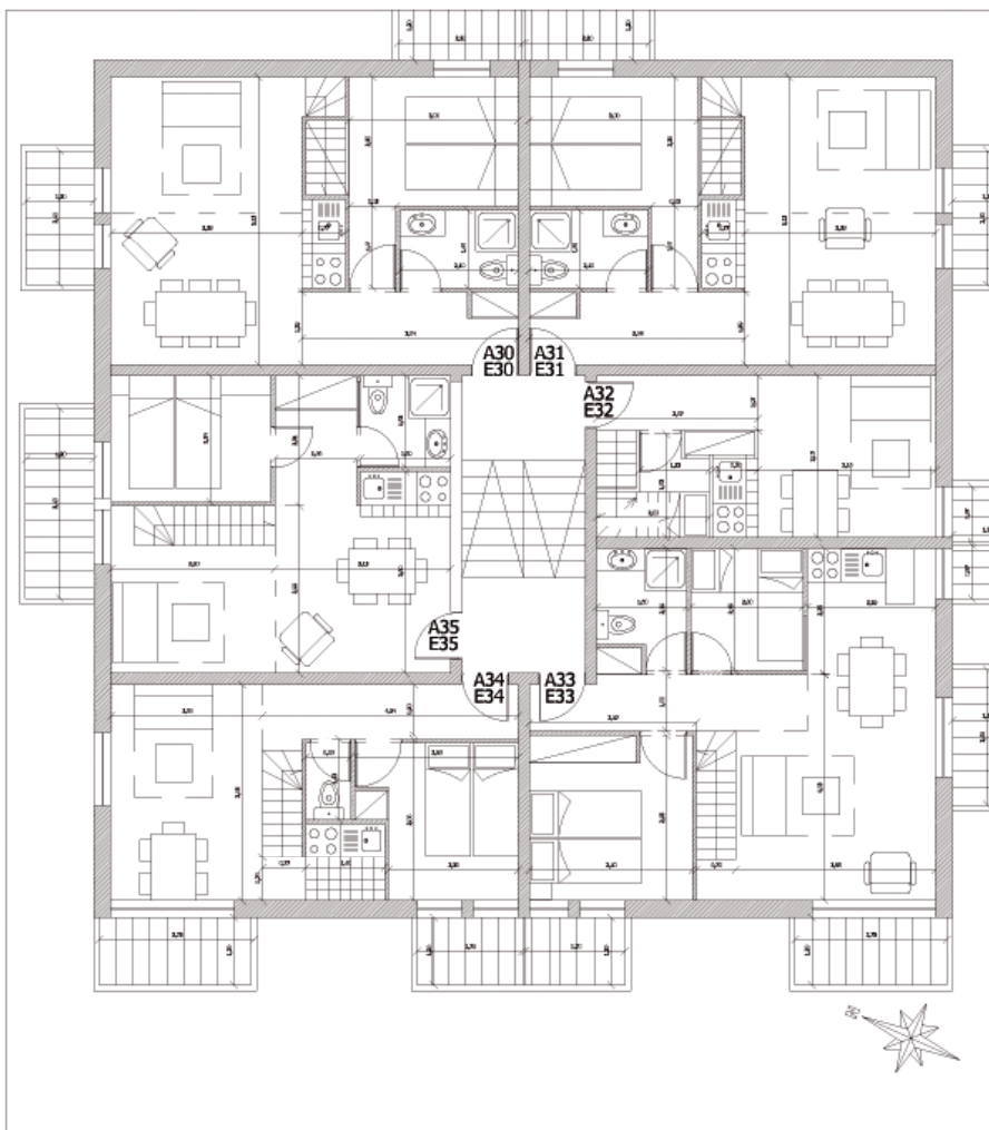
NIVEAU R+3
