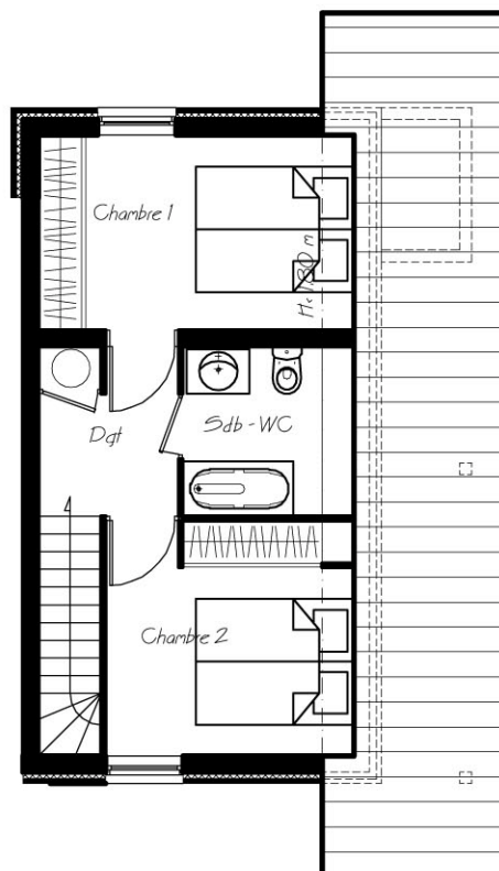
VUE EN PLAN : NIVEAU COMBLES
