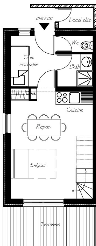
VUE EN PLAN : NIVEAU REZ-DE-CHAUSSEE
