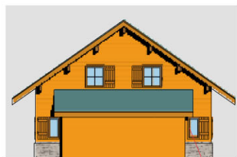
FACADE NORD
