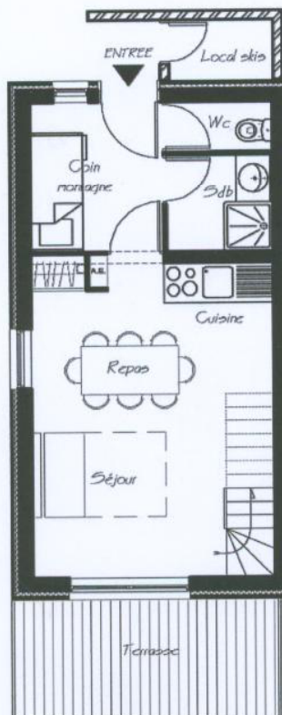
VUE EN PLAN : NIVEAU REZ-DE-CHAUSSÉE
