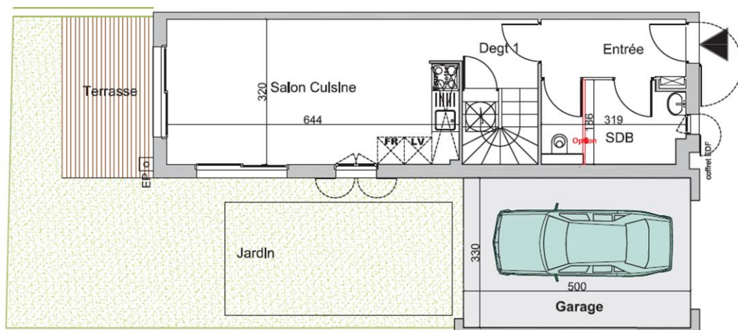
REZ DE CHAUSSE
