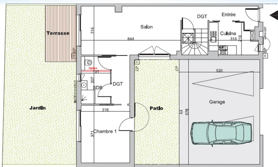
REZ DE CHAUSSE
