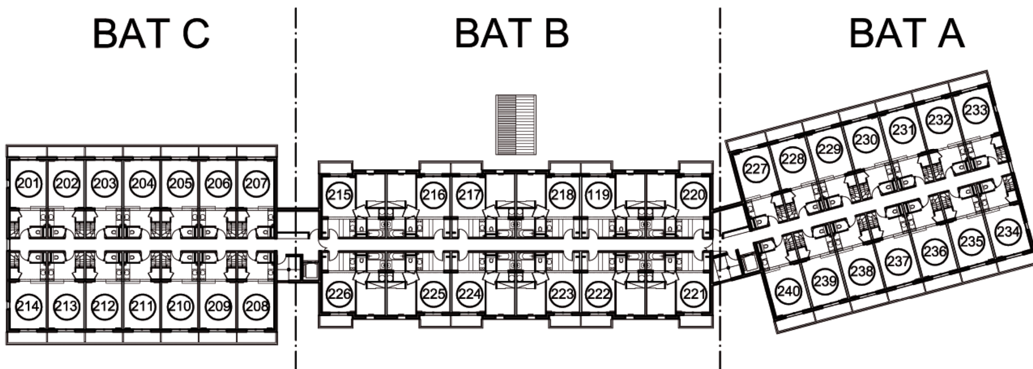
PLAN DU 2° ETAGE
