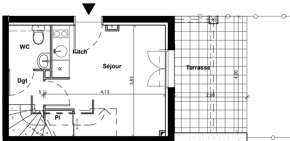
Rez de Jardin
